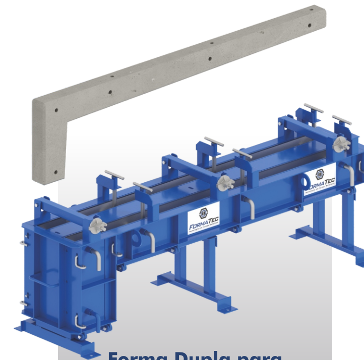
Forma Dupla para Cruzeta tipo "L"
