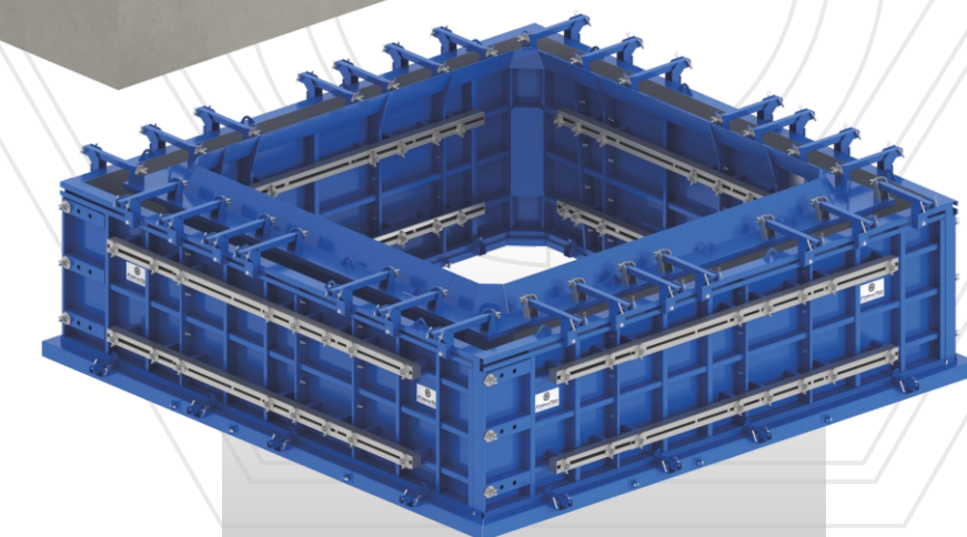
Forma Regulável para Galeria Quadrada
