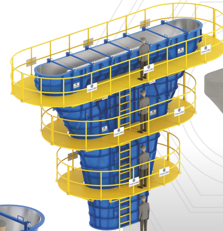
Forma para Capitel concretagem In-Loce
