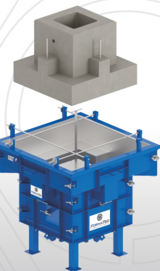
Forma para Sapata com Console Lateral
