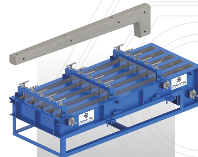
Bateria de Cruzeta tipo "L"
