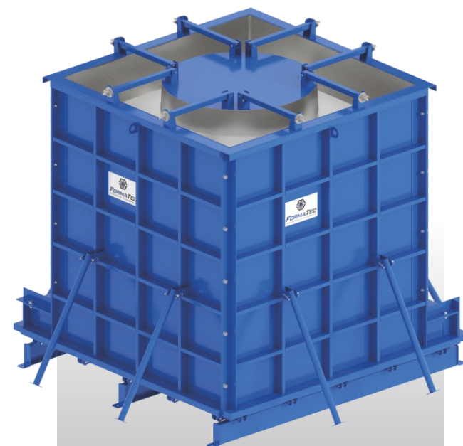
Bloco de Balanço
