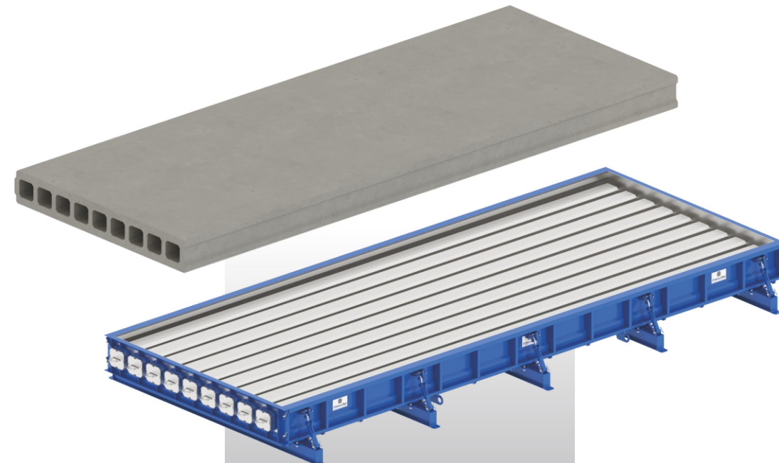
Parede com Alveolos
