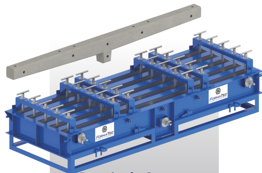
Bateria de Cruzeta tipo "T"
