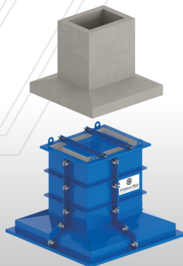
Forma para Sapata
