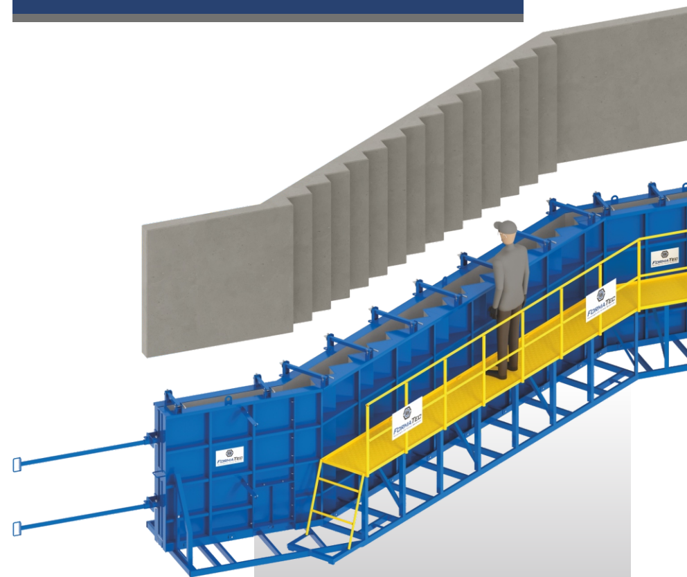
Forma Simples para Escada Pré-Moldada
