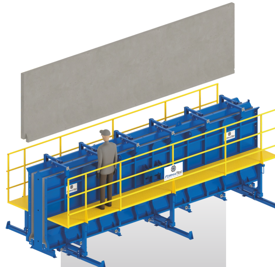
Forma Dupla para Placa de Fechamento com Pingadeira Sistema Deslizante
