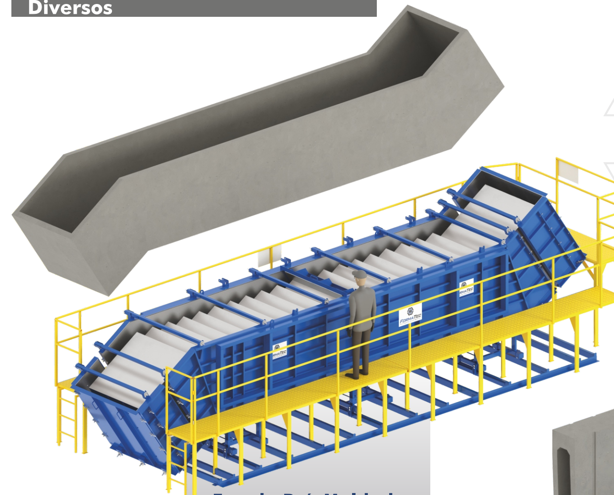
Escada Pré-Moldada com Guarda Corpo
