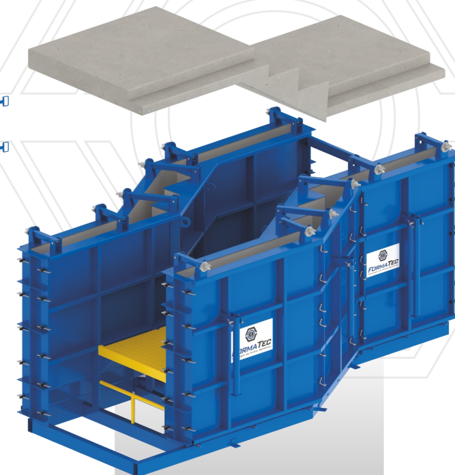
Forma Dupla para Escada Pré-Moldada
