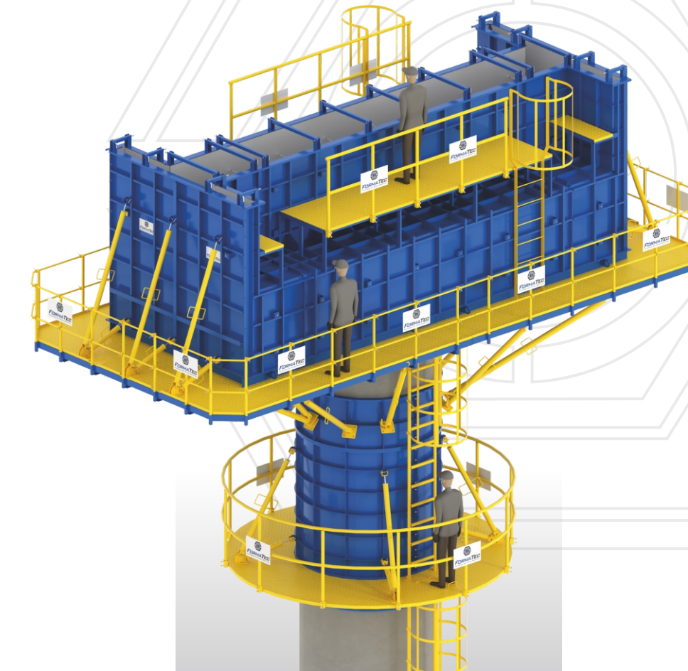
Travessa – Concretagem In-Loco
